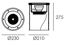
FISSO / FIXED
